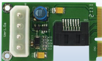
PMMC (mSATA-SATA アダプタ (SATA 電源対応)) x1
